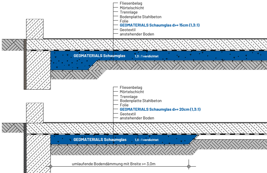
Flächenschüttung einer Industriehalle
